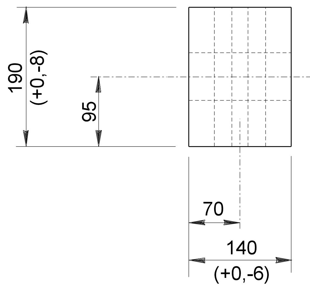
PLAN 1:10
