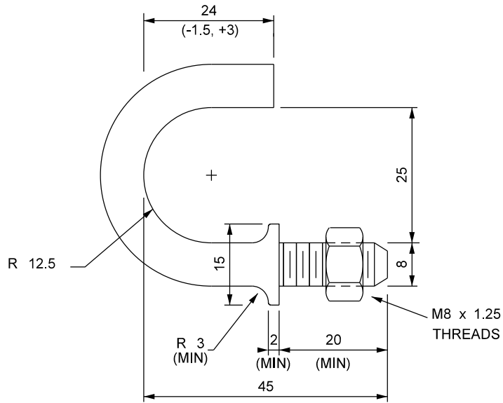
BOLT DETAIL 1:1
