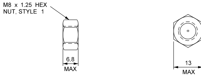
NUT DETAIL 1:1
